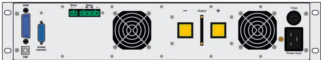
Rückansicht Modell mit 3W-Option
